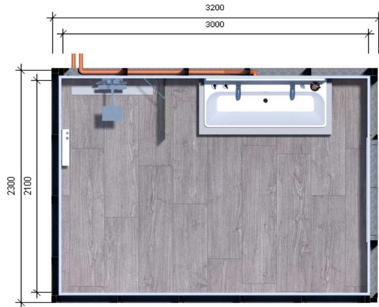
PLATTEGROND
