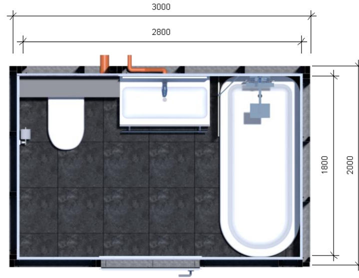
PLATTEGROND
