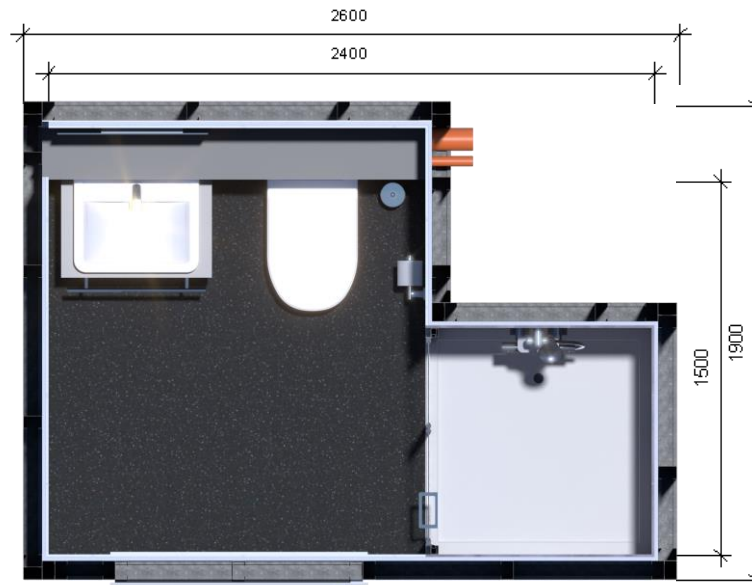
PLATTEGROND
