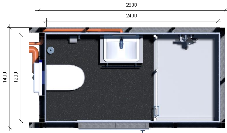
PLATTEGROND
