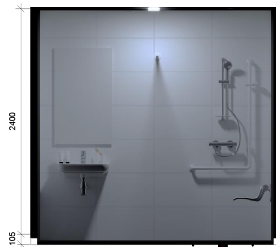
AANZICHT
